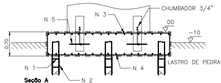
Seção A
