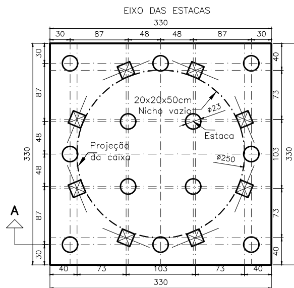
PLANTA
