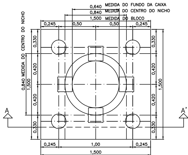
PLANTA escala 1:25
