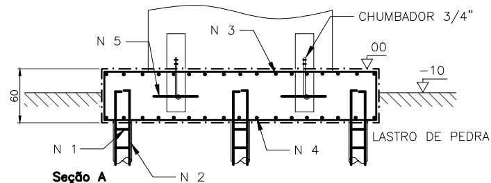
Seção A
