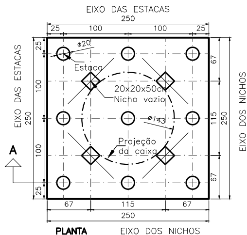
PLANTA
